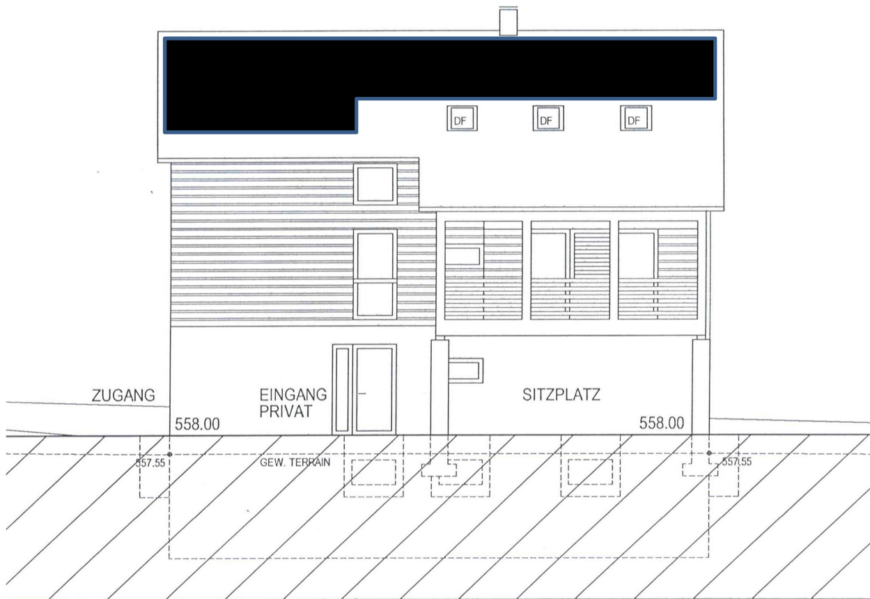
NORDWESTFASSADE
