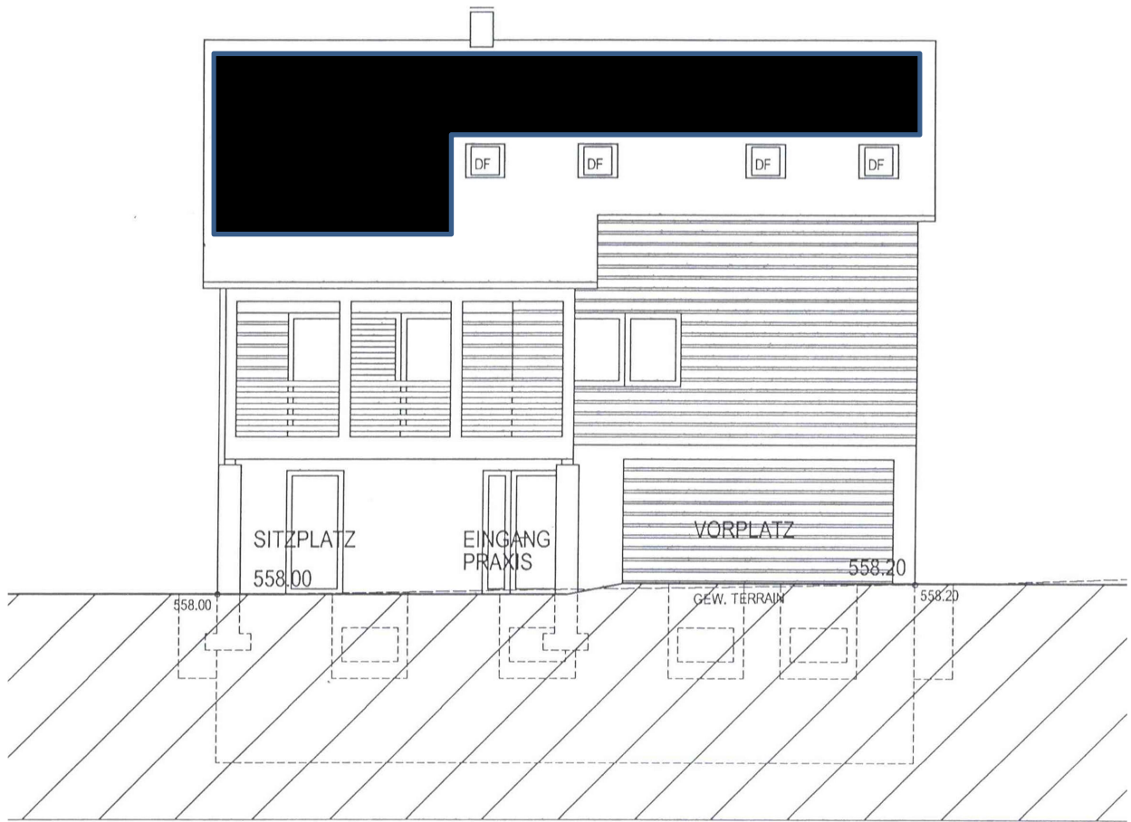
SÜDOSTFASSADE
